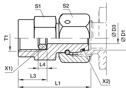
X1) Уплотн. кольцо DK1 X2) Уплотн. кольцо OR
