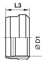
Прогрессивное кольцо: DPR
