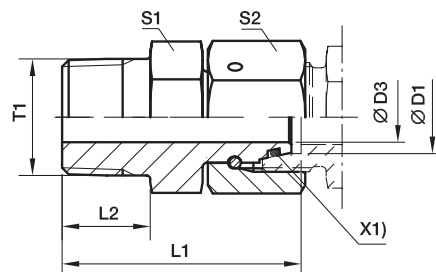
X1) Уплотн. кольцо OR
