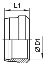
Врезное кольцо: D-образное
