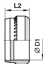
Стопорное кольцо: PSR
