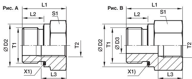
X1) Уплотнитель Eolastic ED
