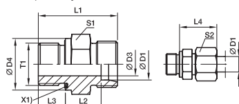
X1) Уплотнитель Eolastic ED
