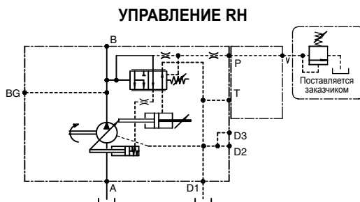
РАСПОЛОЖЕНИЕ ПРОТИВ ЧАСОВОЙ СРЕЛКИ Показан P*075
