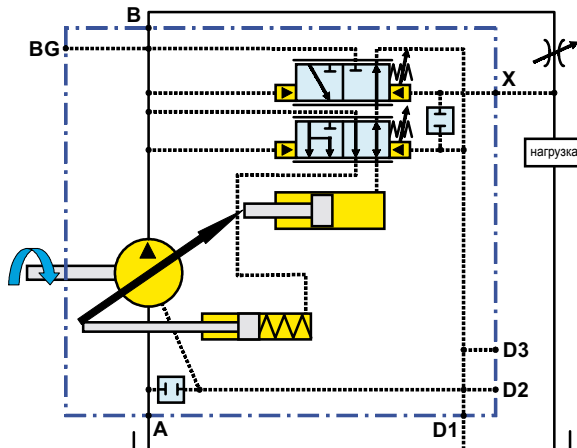
схематическая диаграмма
