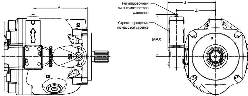
РАСПОЛОЖЕНИЕ ПО ЧАСОВОЙ СТРЕЛКЕ Показан Р*075
