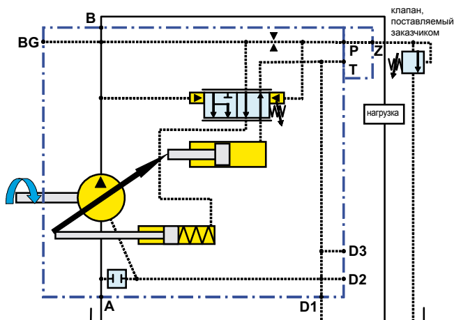
«RH» Сервоуправление
