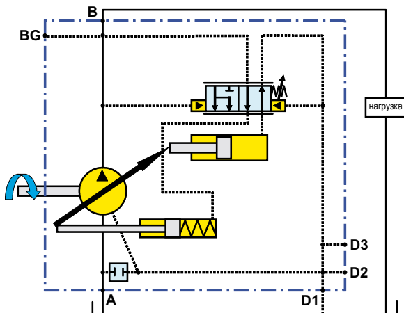
Управление с ограничителем давления
