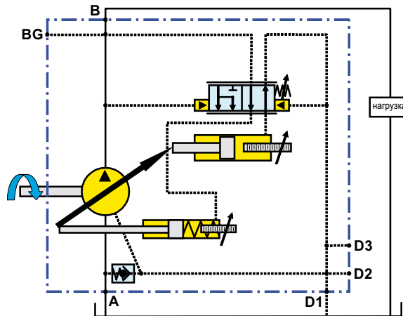
Управление с ограничителем давления с дополнительной регулировкой минимального и максимального рабочего объема и обратным клапаном между корпусом и линией всасывания (Для ограничения минимального рабочего объема необходим клапан сброса в системе.)
